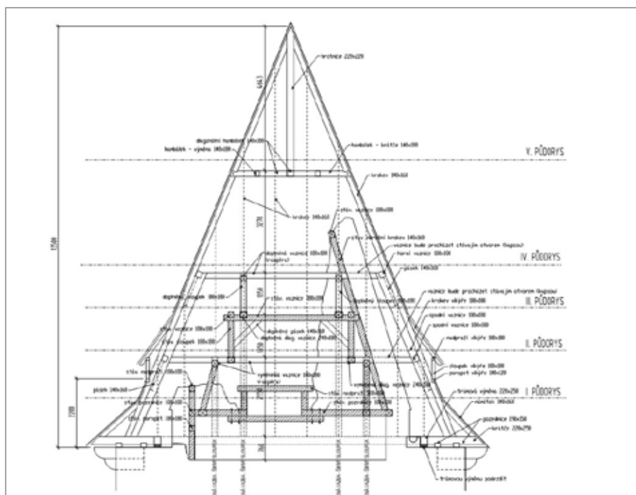
Projekt nového zastřešení (foto: archiv hradu)
